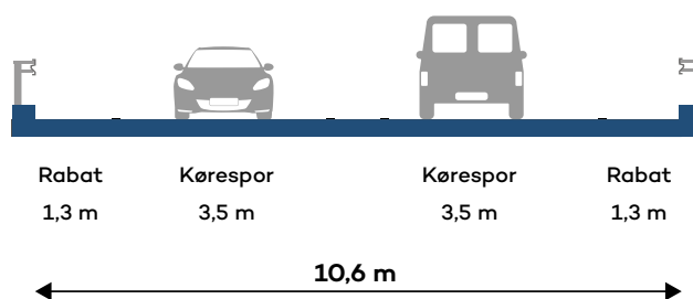
Figur 3.1 Eksempel på 2-sporet tværsnit i broløsninger.
