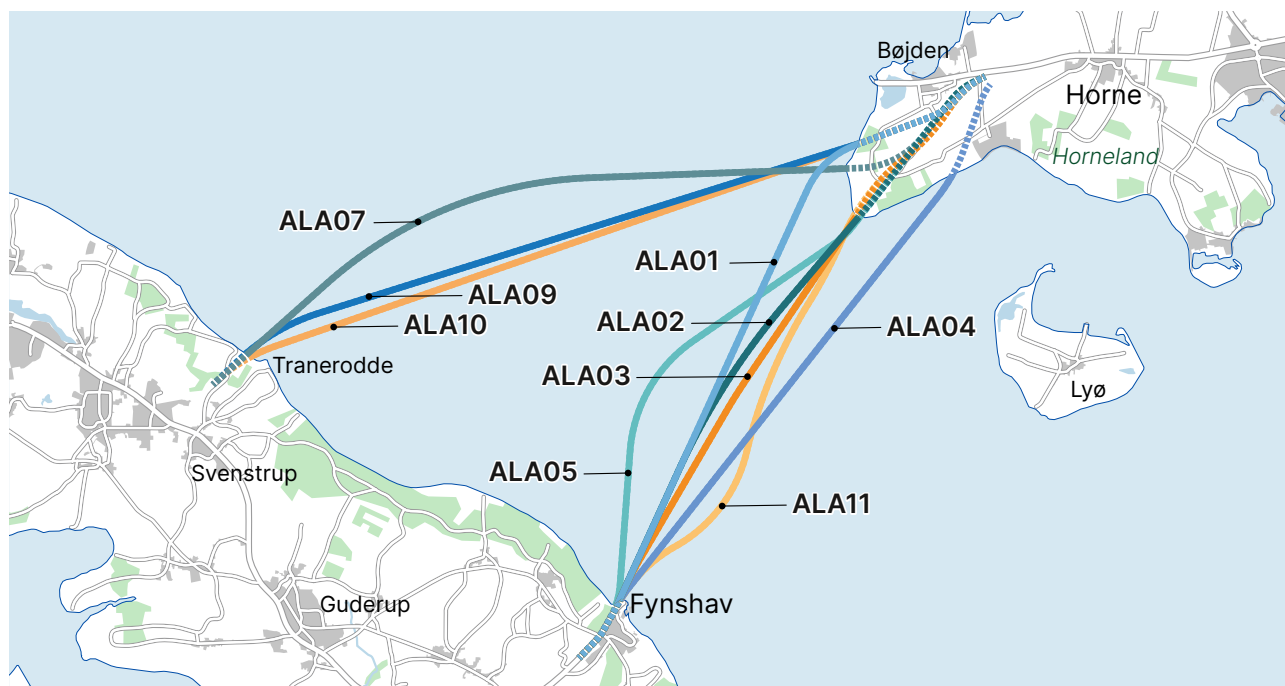
Figur 3.9 De 9 undersøgte korridorer.
