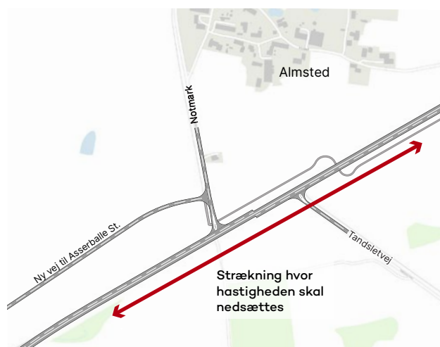
Figur 4.7 Ved Almsted nedsættes hastigheden over en strækning på ca. 650 meter ved krydset med forskudte sideveje.
