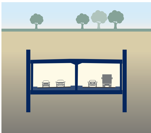
Gravet tunnel, principskitse.
