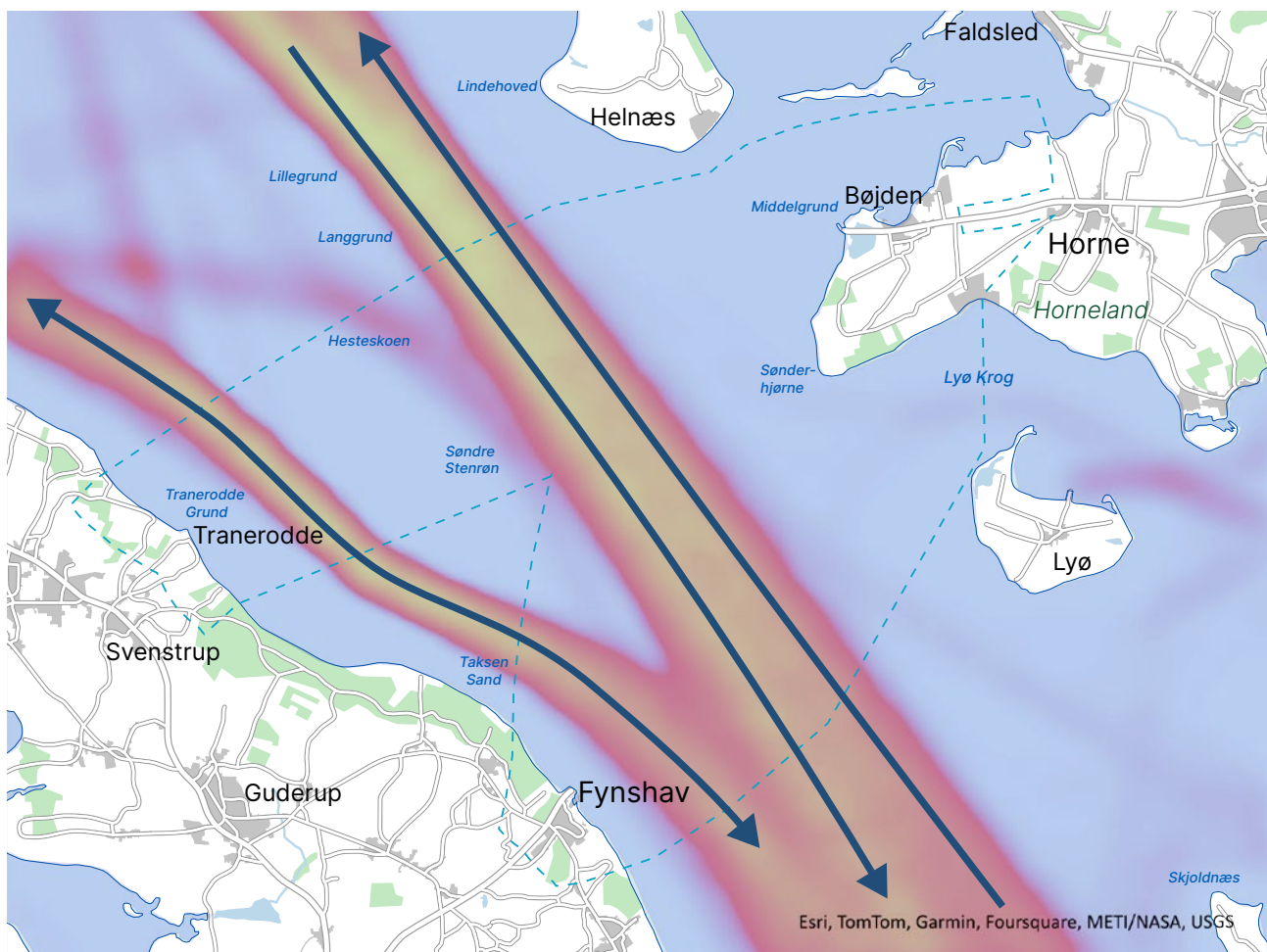
Figur 3.2 Trafikæthedskort for fragt- og tankskibe i 2021.
