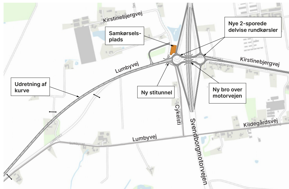
Figur 4.13 Ombygning af tilslutningsanlæg 11 ved Årslø.
