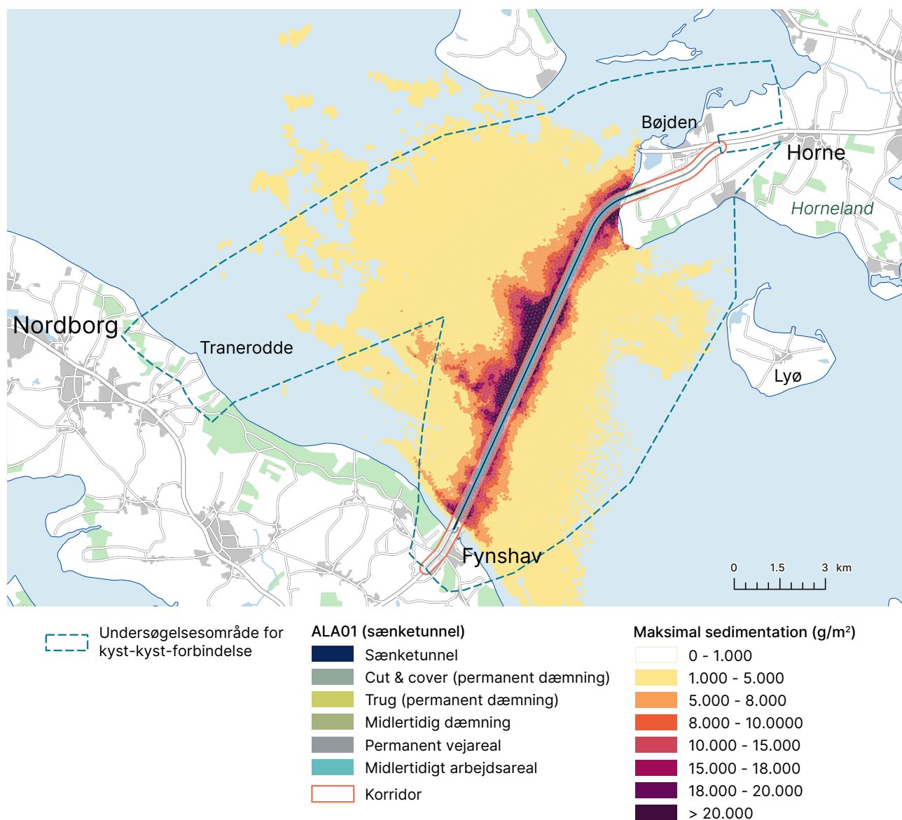
Figur 3.17 Den maksimale koncentration af frigivne sedimenter ved uddybning af tunnelrende til sænkettunnelen ALA01. Kvælstof frigives fra disse sedimenter.
