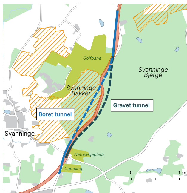
Figur 4.11 Undersøgte tunnelloøsninger ved Svanning Bakker.
