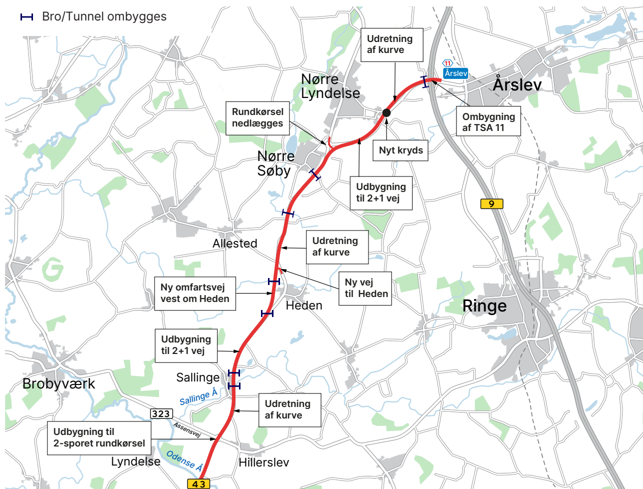
Figur 4.12 Udbygning på den nordlige vejstrækning på Fyn.
