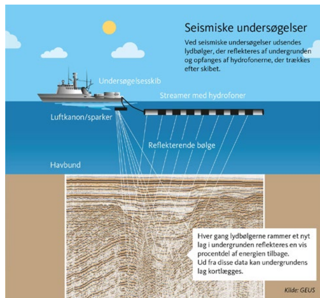
Figur 3.3 Seismiske undersøgelser.
