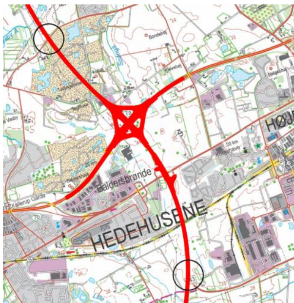
Figur 4-4: Tilslutningsanlæg og forbindelsesanlæg ved Høje Taastrup. Kilde: Snit fra tegning 93010-1066
